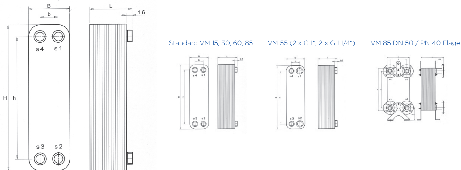
Esquema : Dimensões
