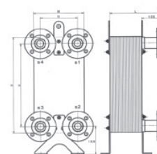
VM 85 DN 50 / PN 40 Flange
