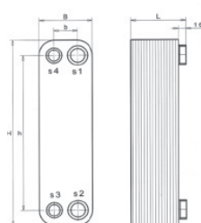
VM 55 (2 x G 1"; 2 x G 1 1/4")
